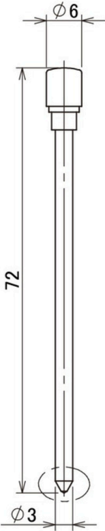
Long Pin
